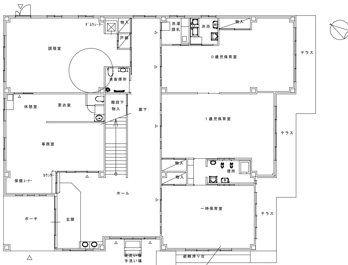
一階平面図
