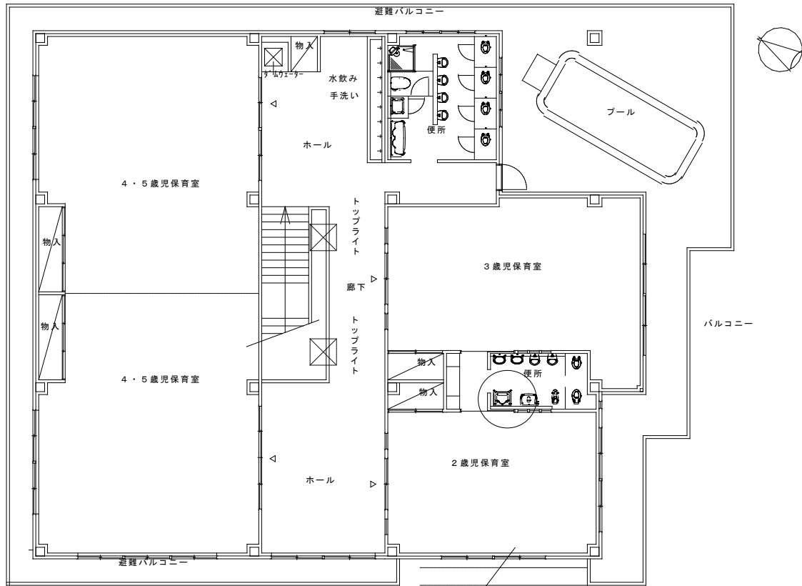
二階平面図
